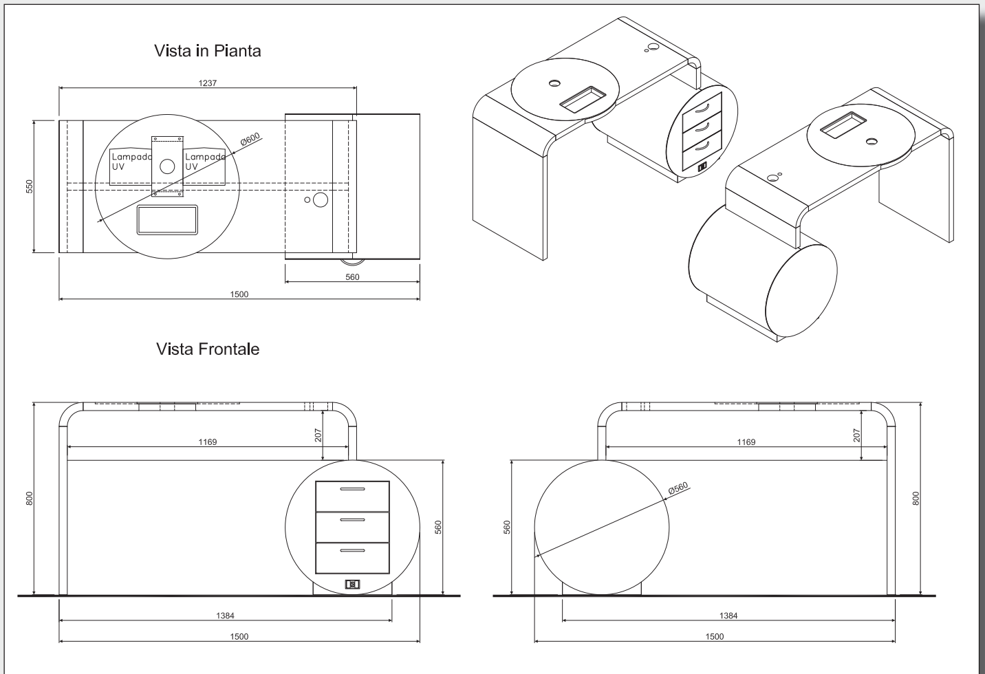
Banco da lavoro WNS-TUBE
